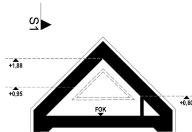
Schnitt 2
