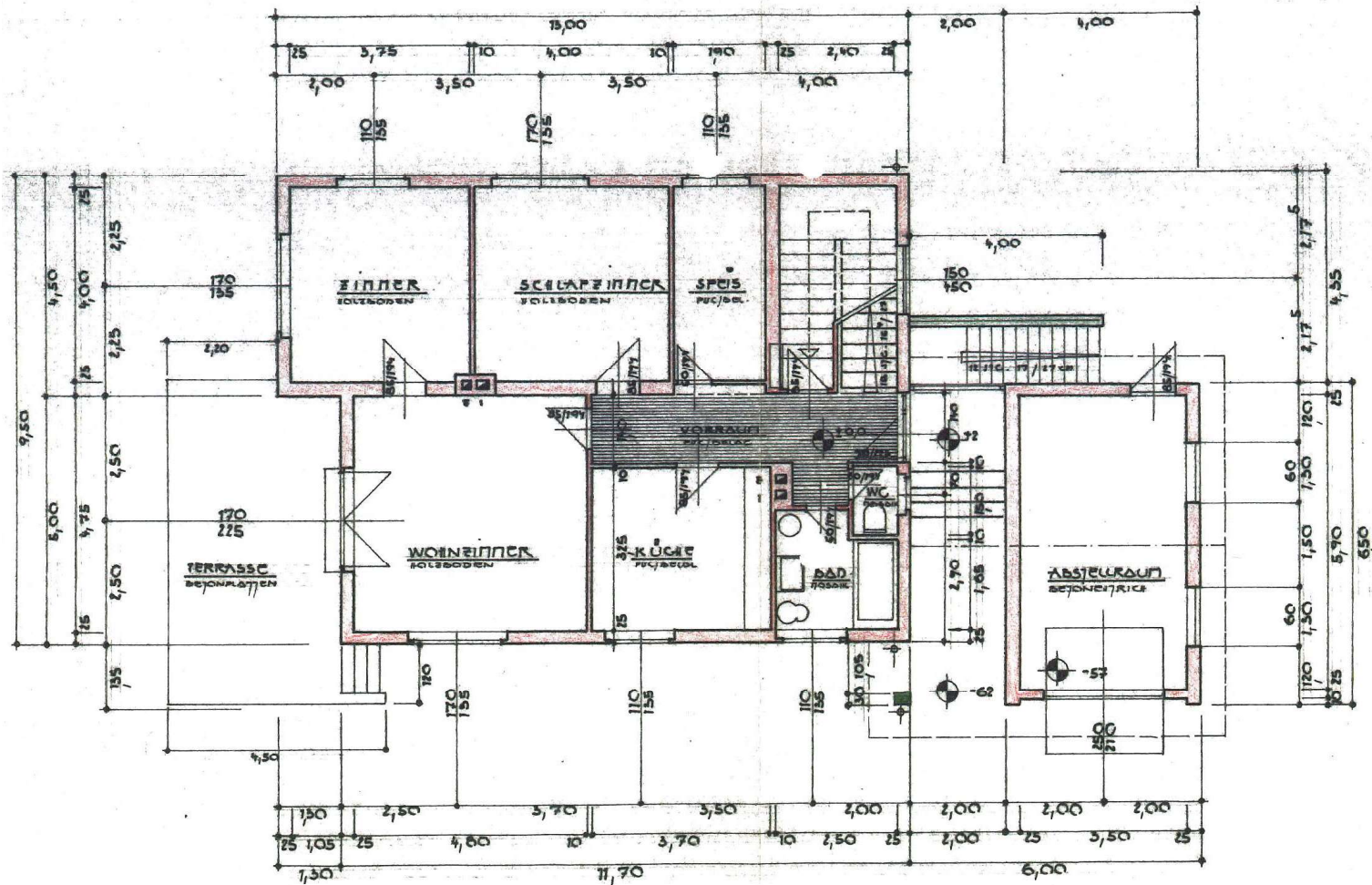
ERDGESCHOSS I
