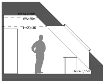
SCHNITT B
