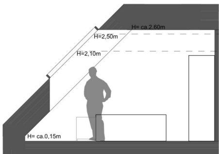
SCHNITT A
