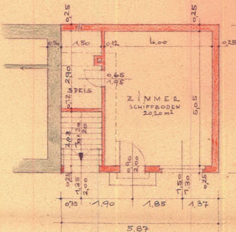
ERDGESCHOSS
