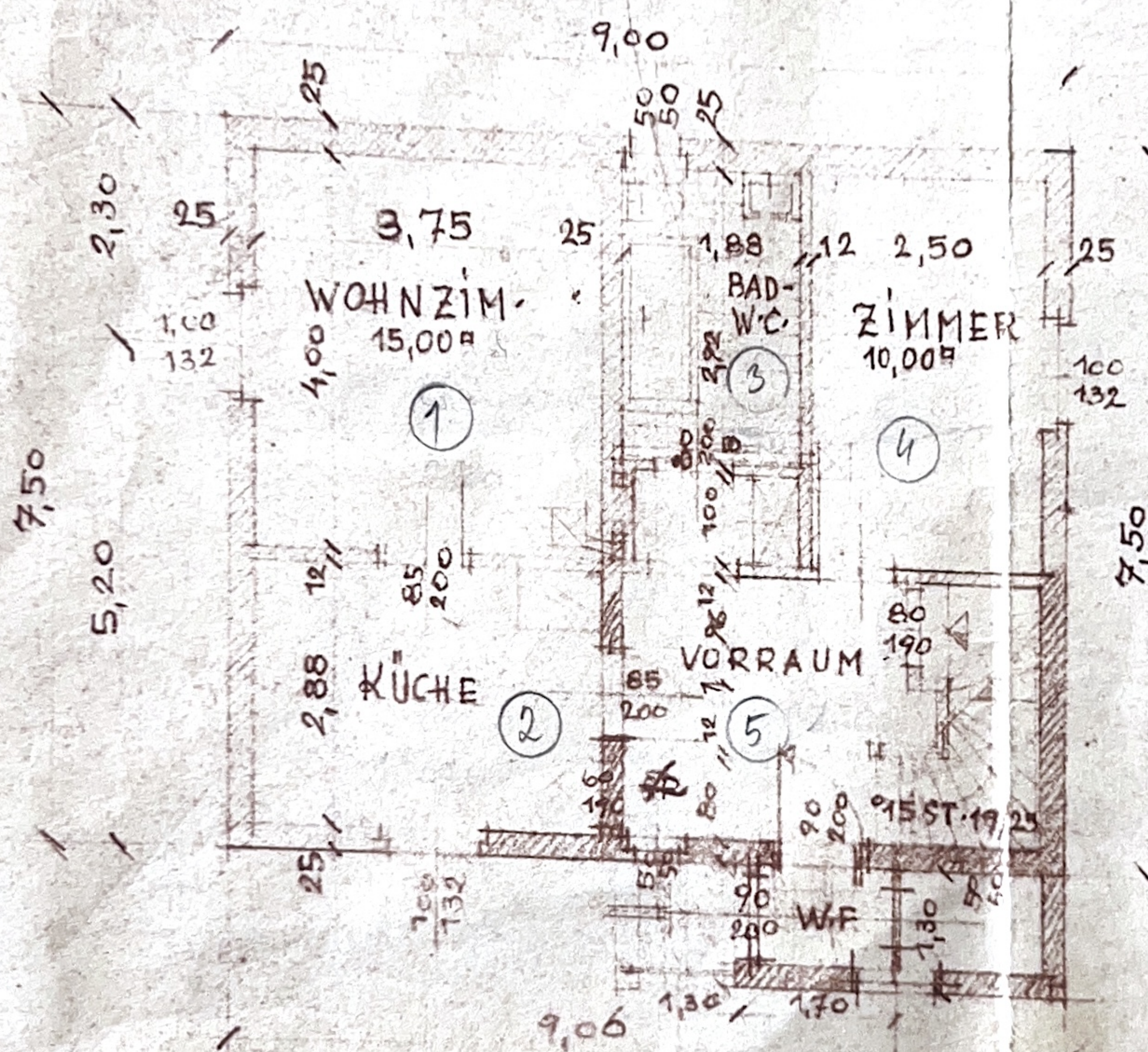
ERDGESCHOSSGRUNDRISS
