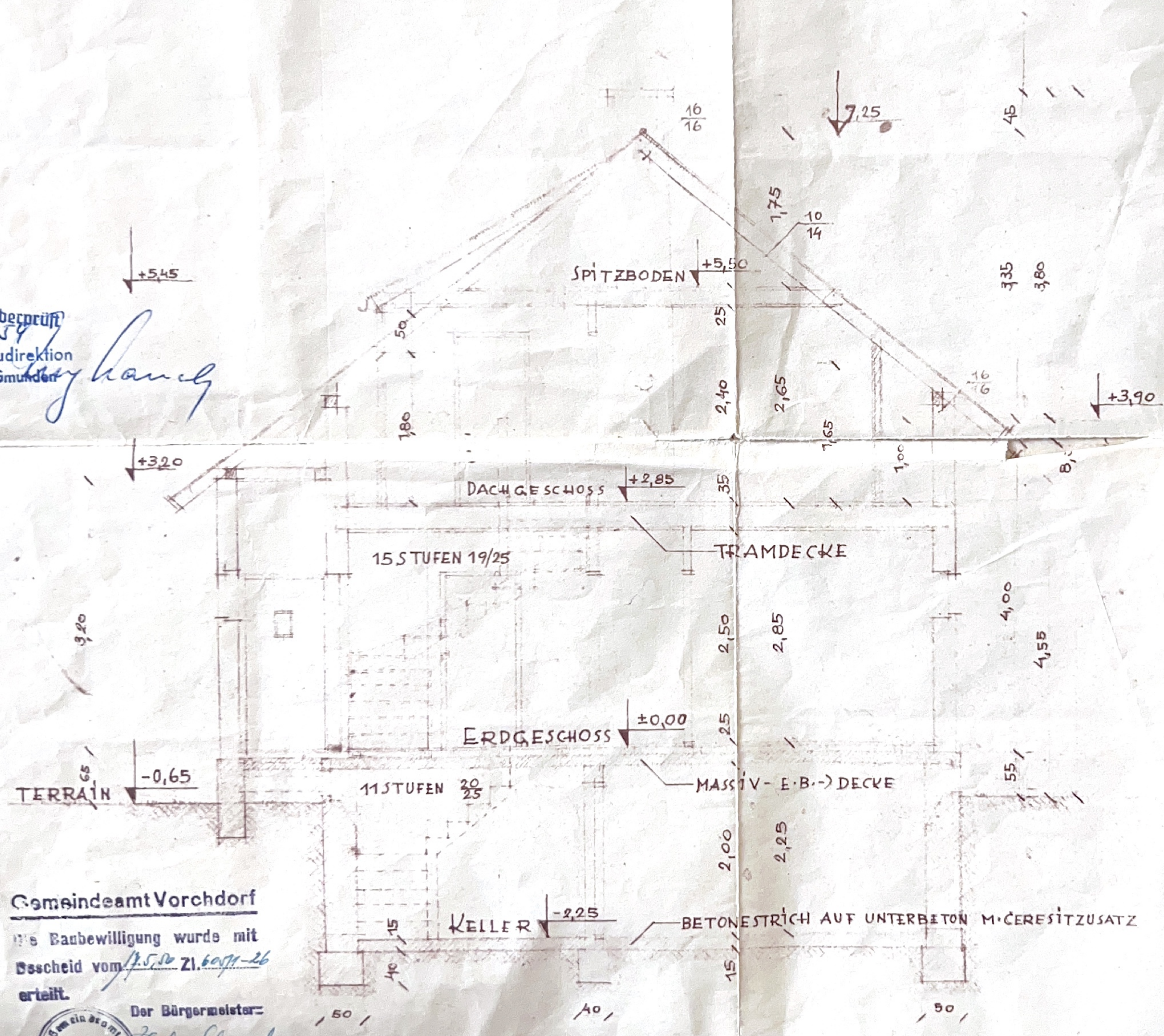
QUERSCHNITT 1:50
