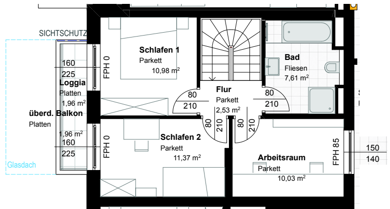
Grundriss 1. OG
