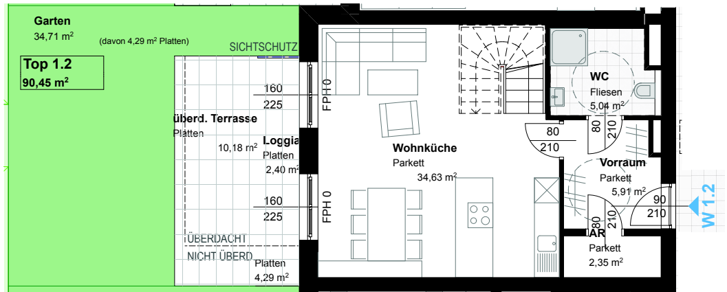
Grundriss GartenG
