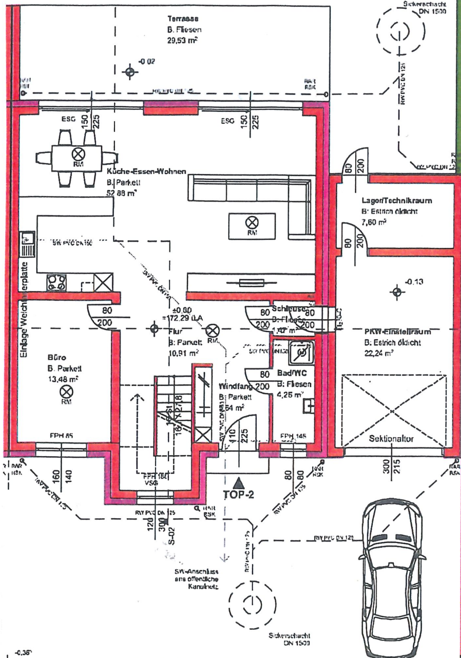
Grundriss EG WNF: 88,63 m 2 M 1:100
