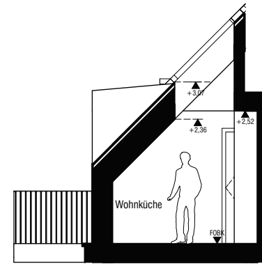
Schnitt
