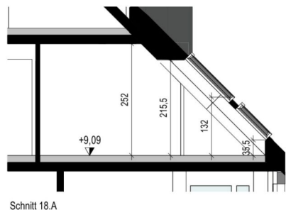
Schnitt 18.A
