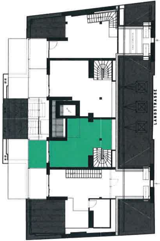
ÜBERSICHT GALERIEGESCHOSS
