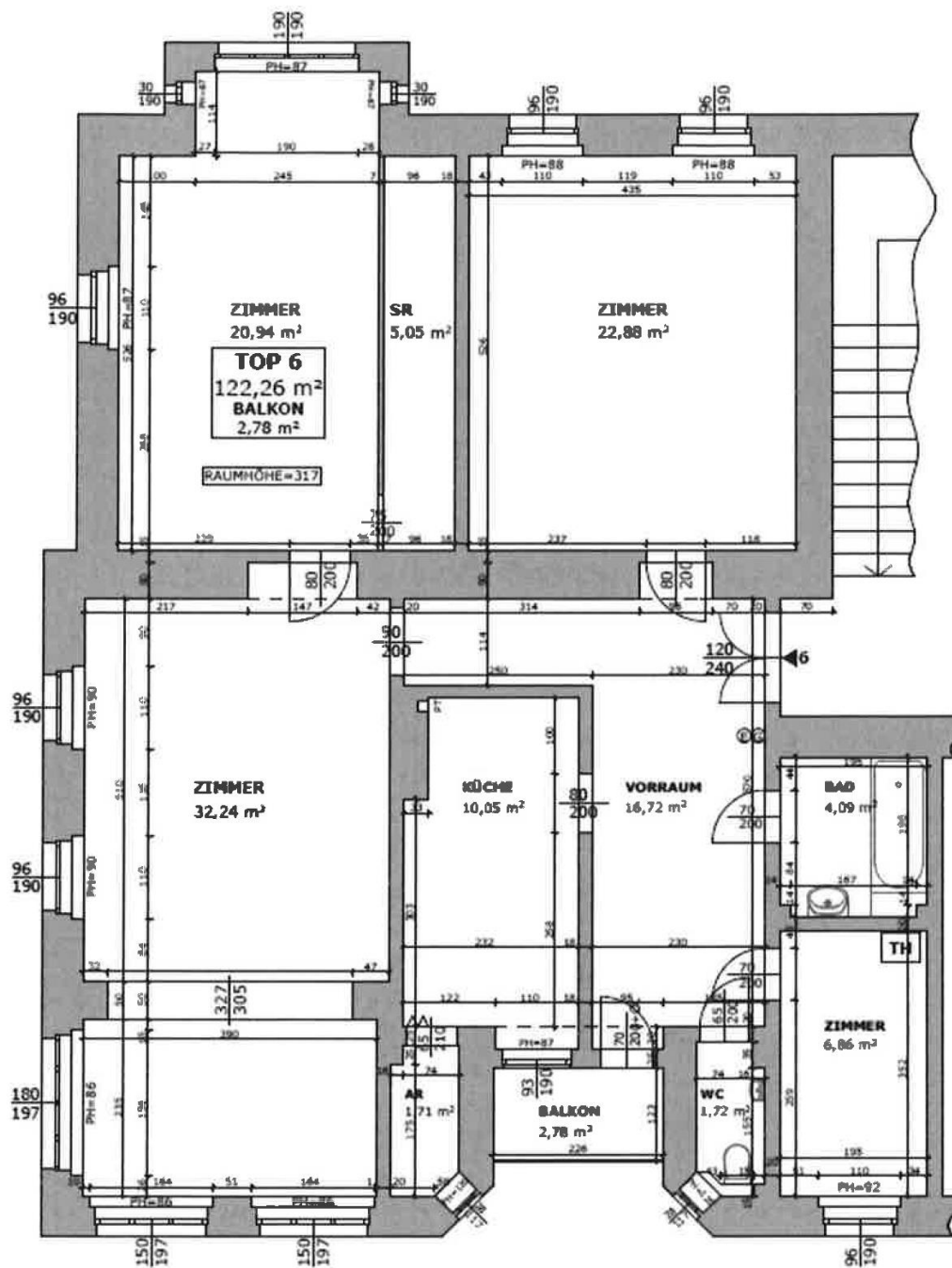
GRUNDRISS 2. STOCK TOP 6
