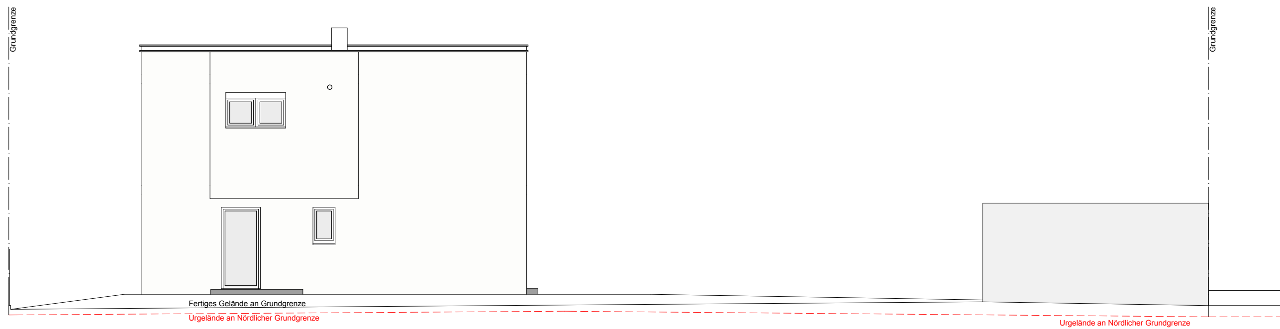
NORD ANSICHT
