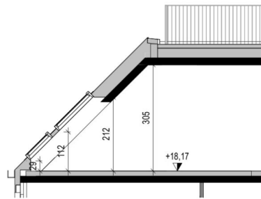
Schnitt 31.A
