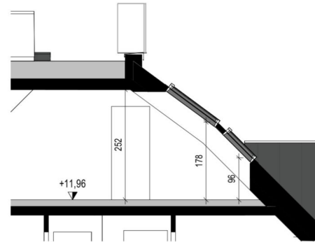
Schnitt 20.C
