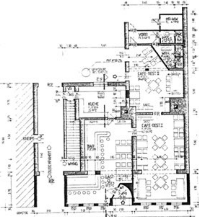
grundriß 1:100 neubau
