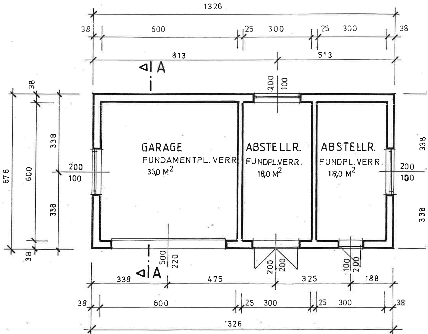
GRUNDRISS
