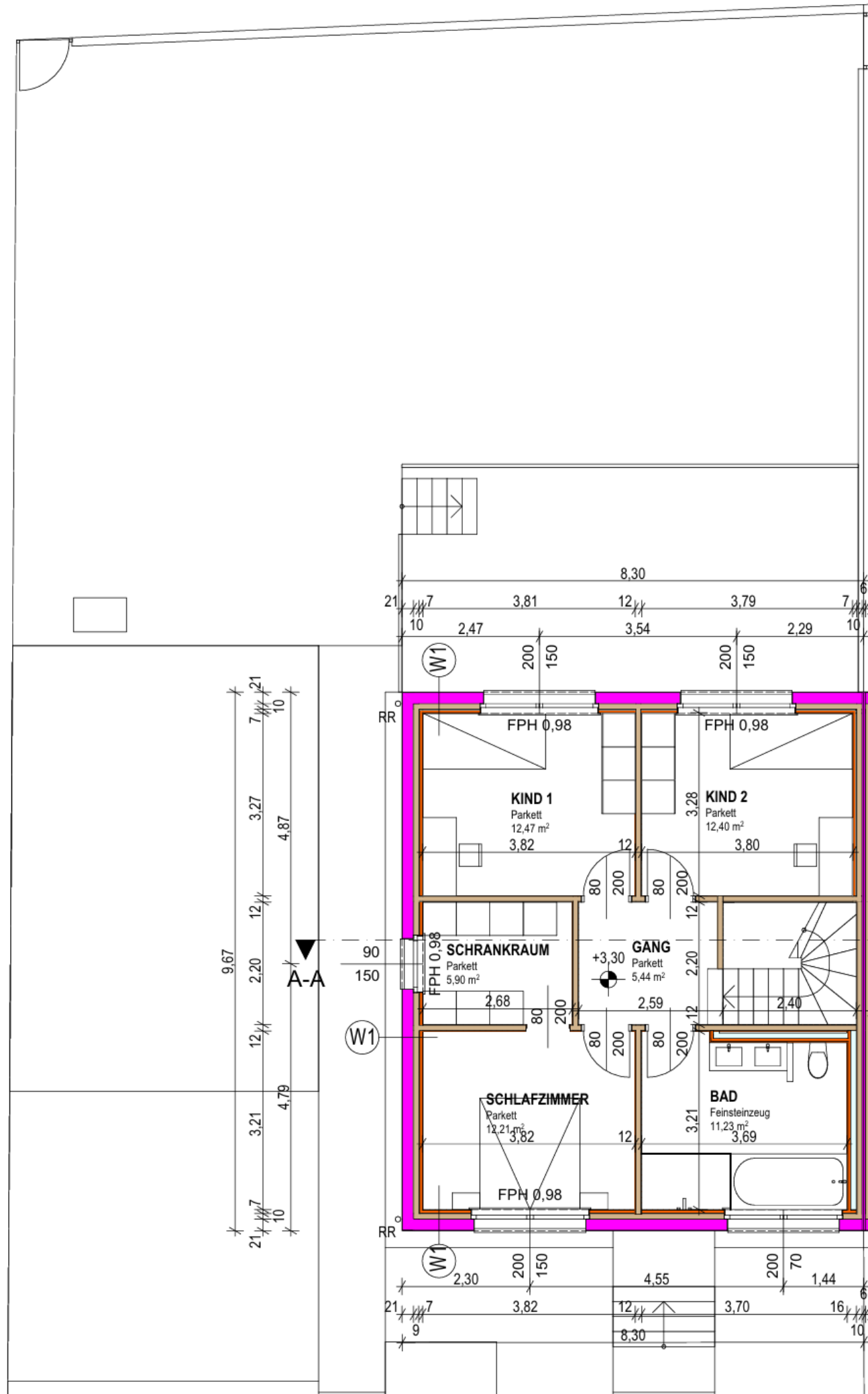
OBERGESCHOSS M1:100
