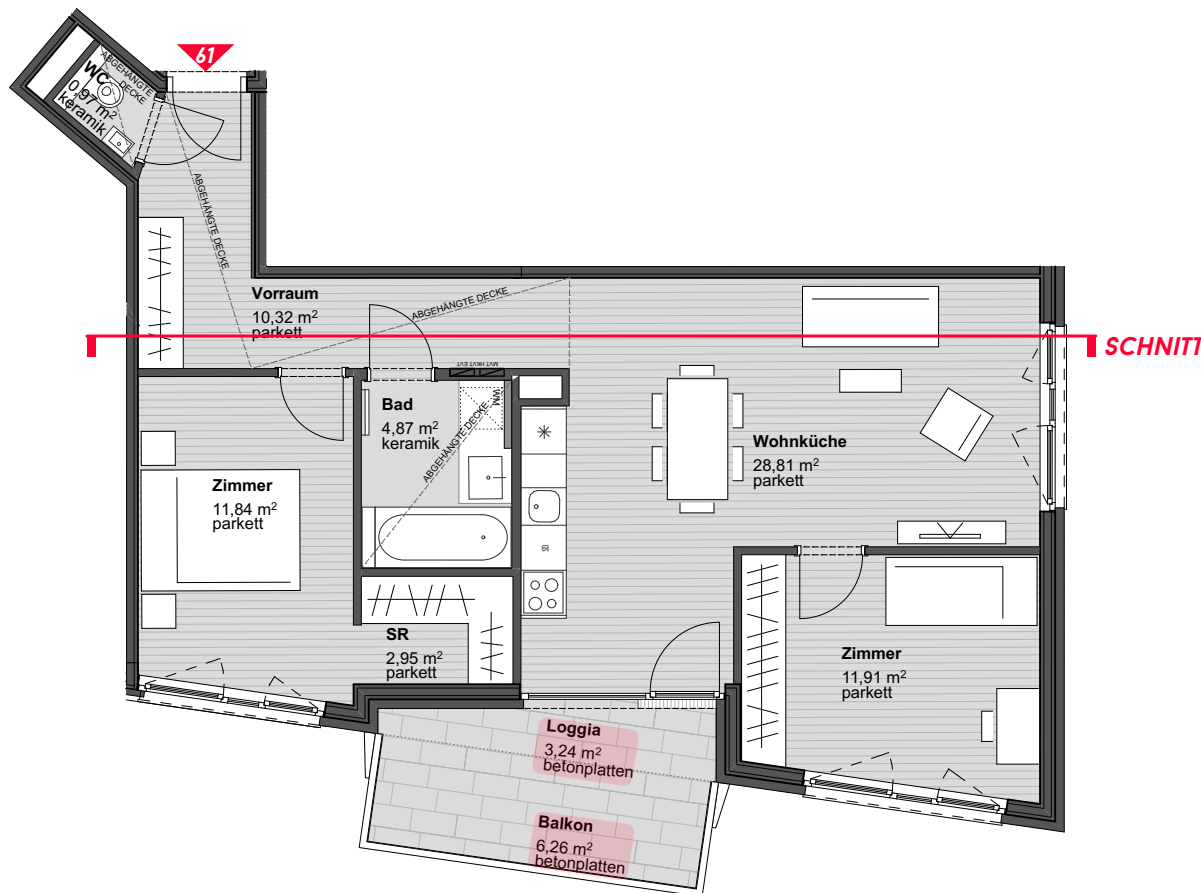
Grundriss | M 1:100
