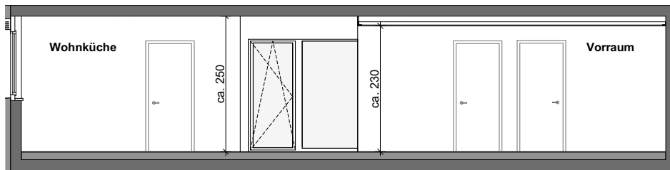
Schnitt | M 1:100
