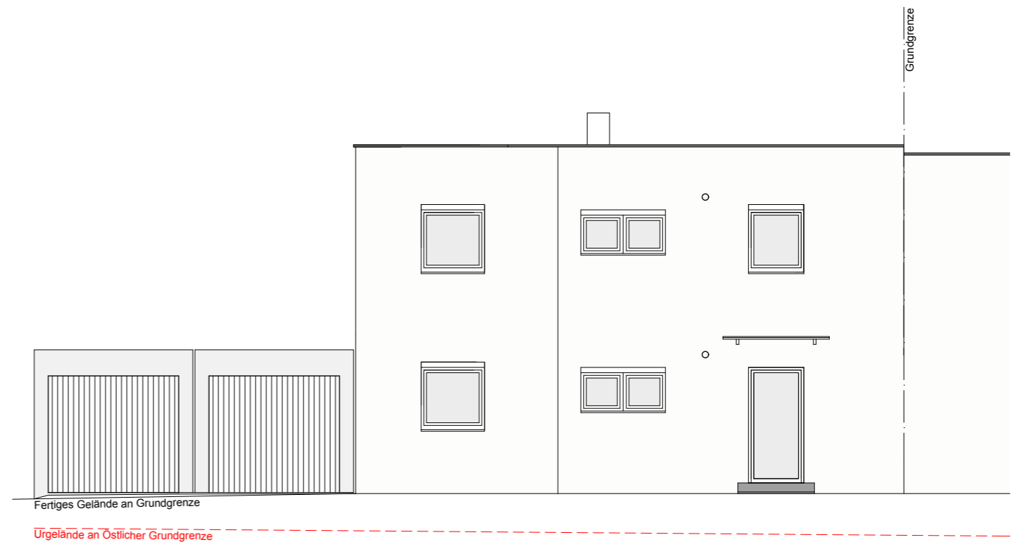
OST ANSICHT
