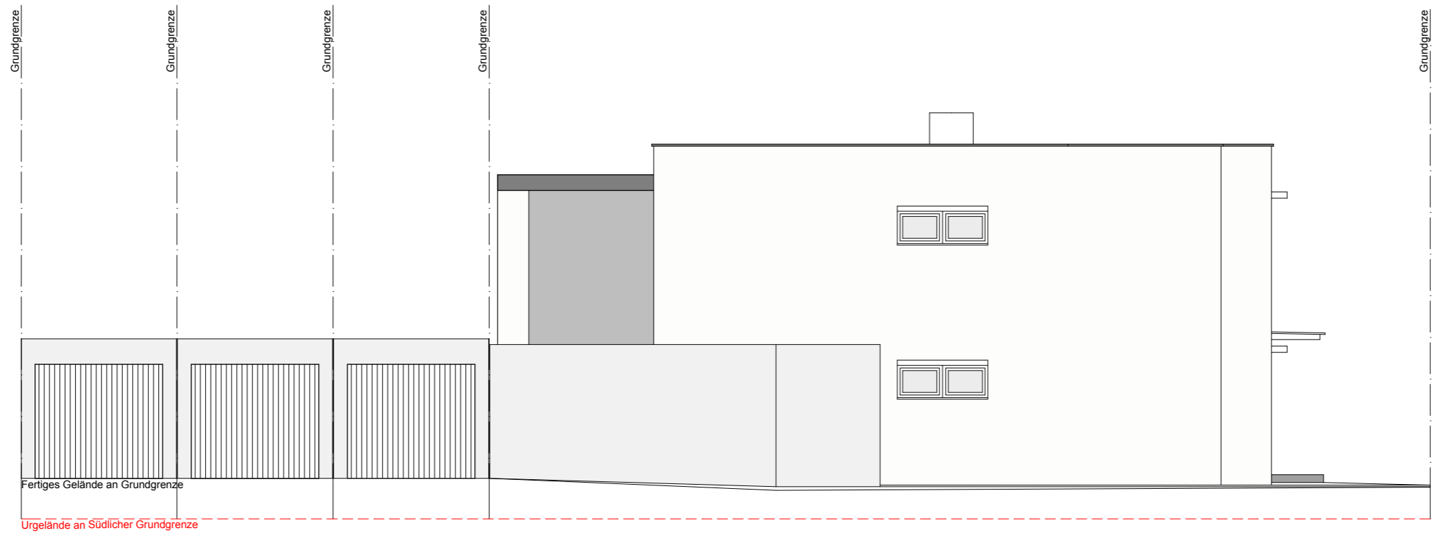
SÜD ANSICHT
