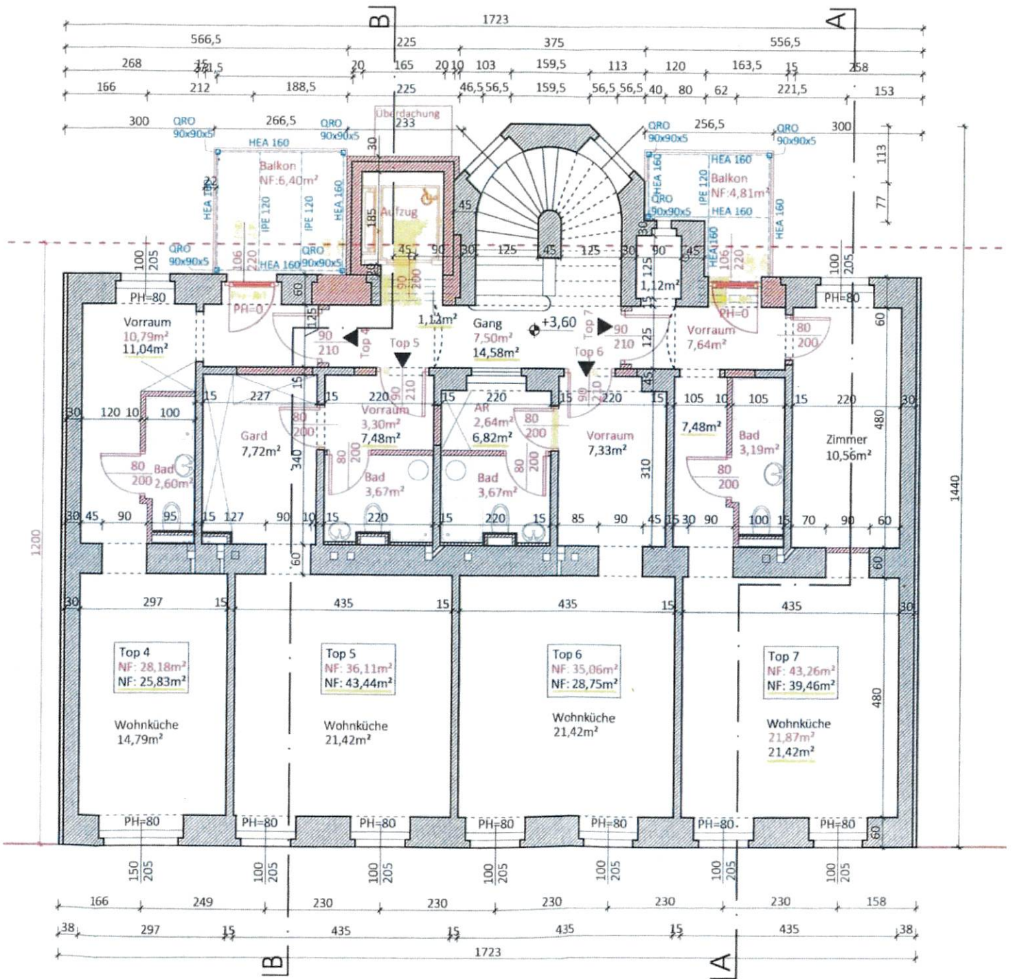
Grundriss 1.Obergeschoss
