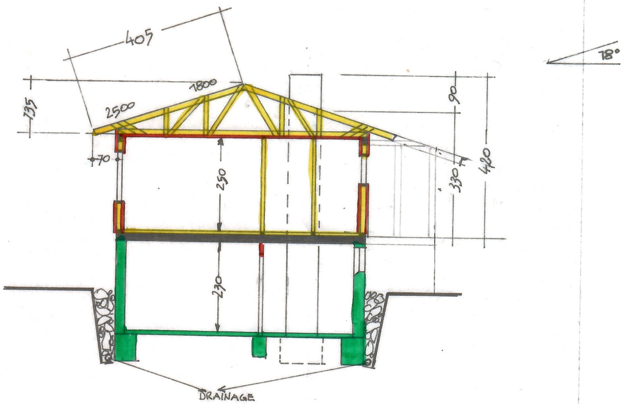
SCHNITT A-B
