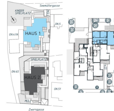
LAGEPLAN
