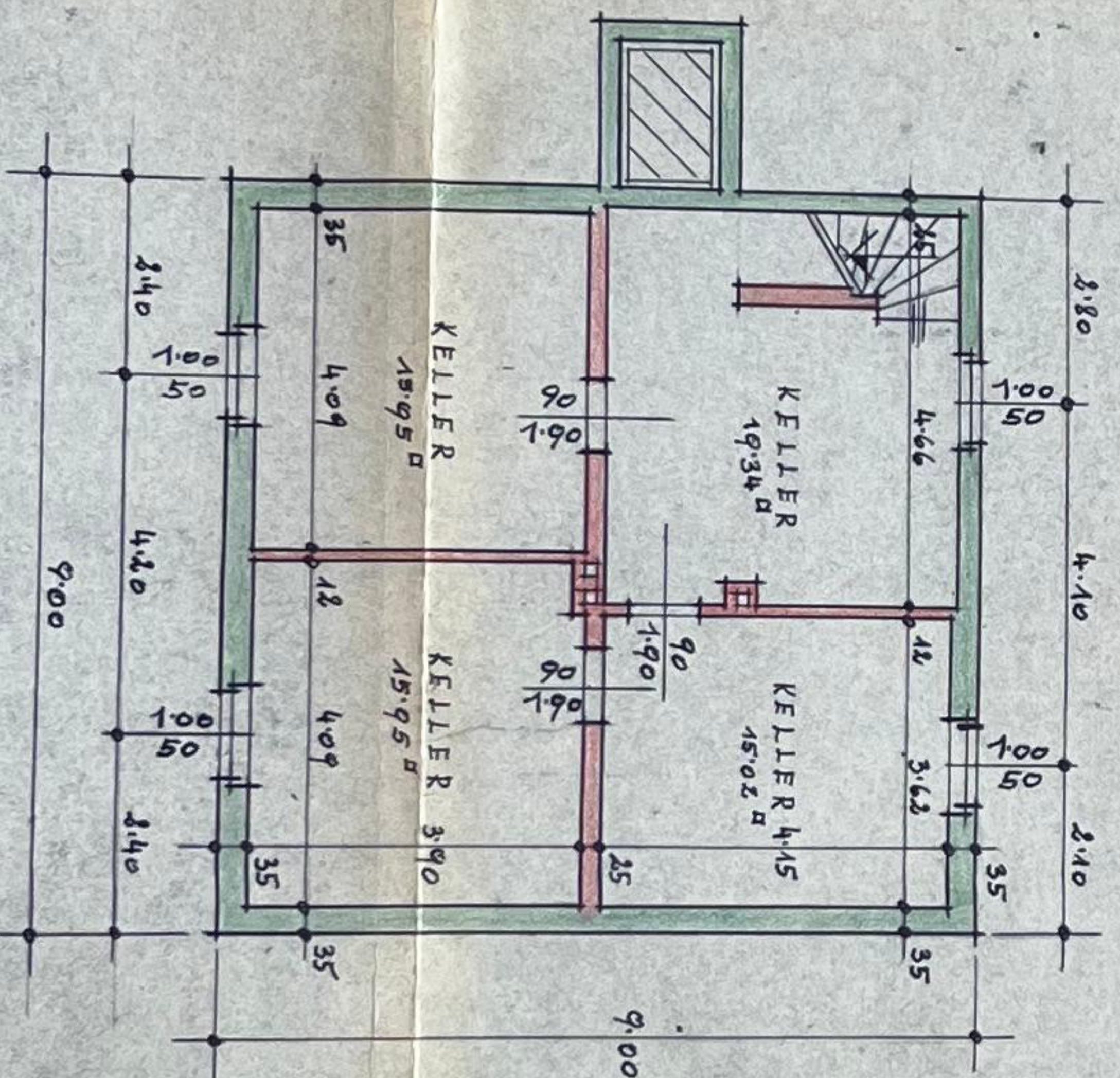
KELLERGESCHOSS
