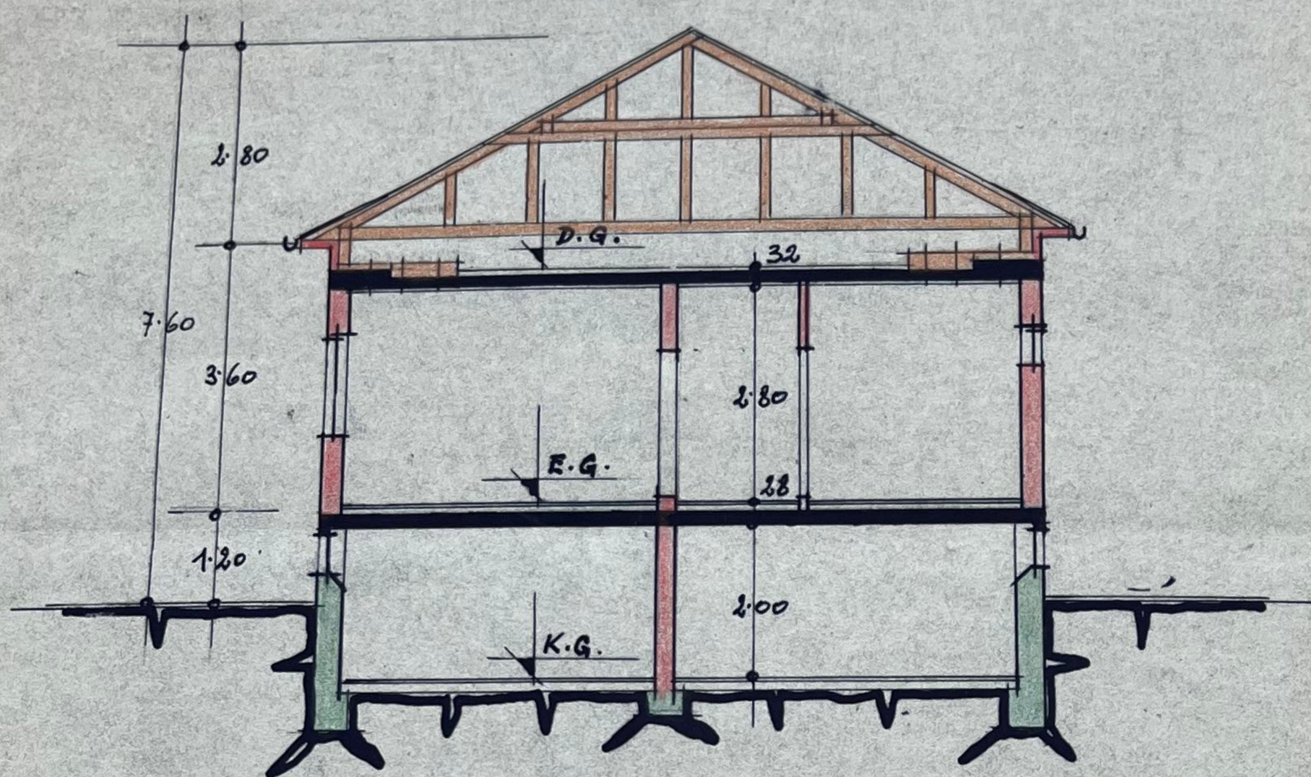
SCHNITT-A-B
