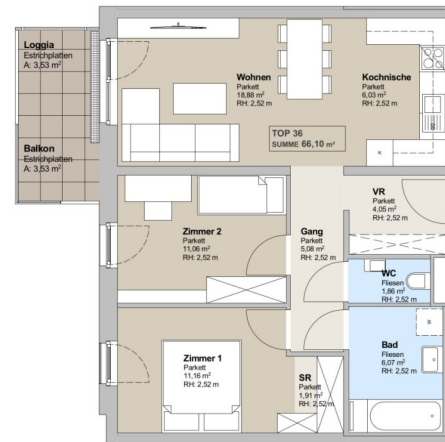
2. Obergeschoù M: 1: 100
