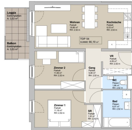
3. Obergeschoù M: 1: 100
