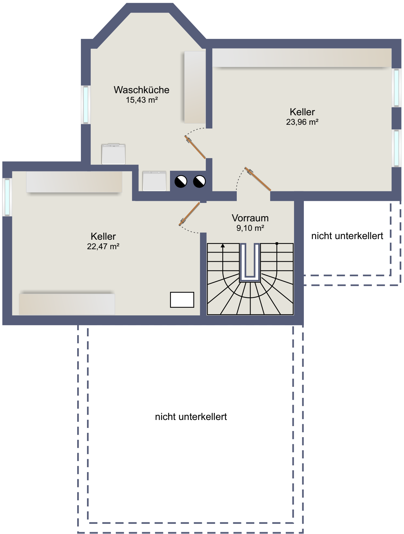
Kellergeschoss
