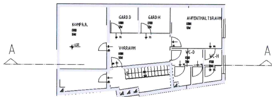
GRUNDRISS OBERGESCHOSS
