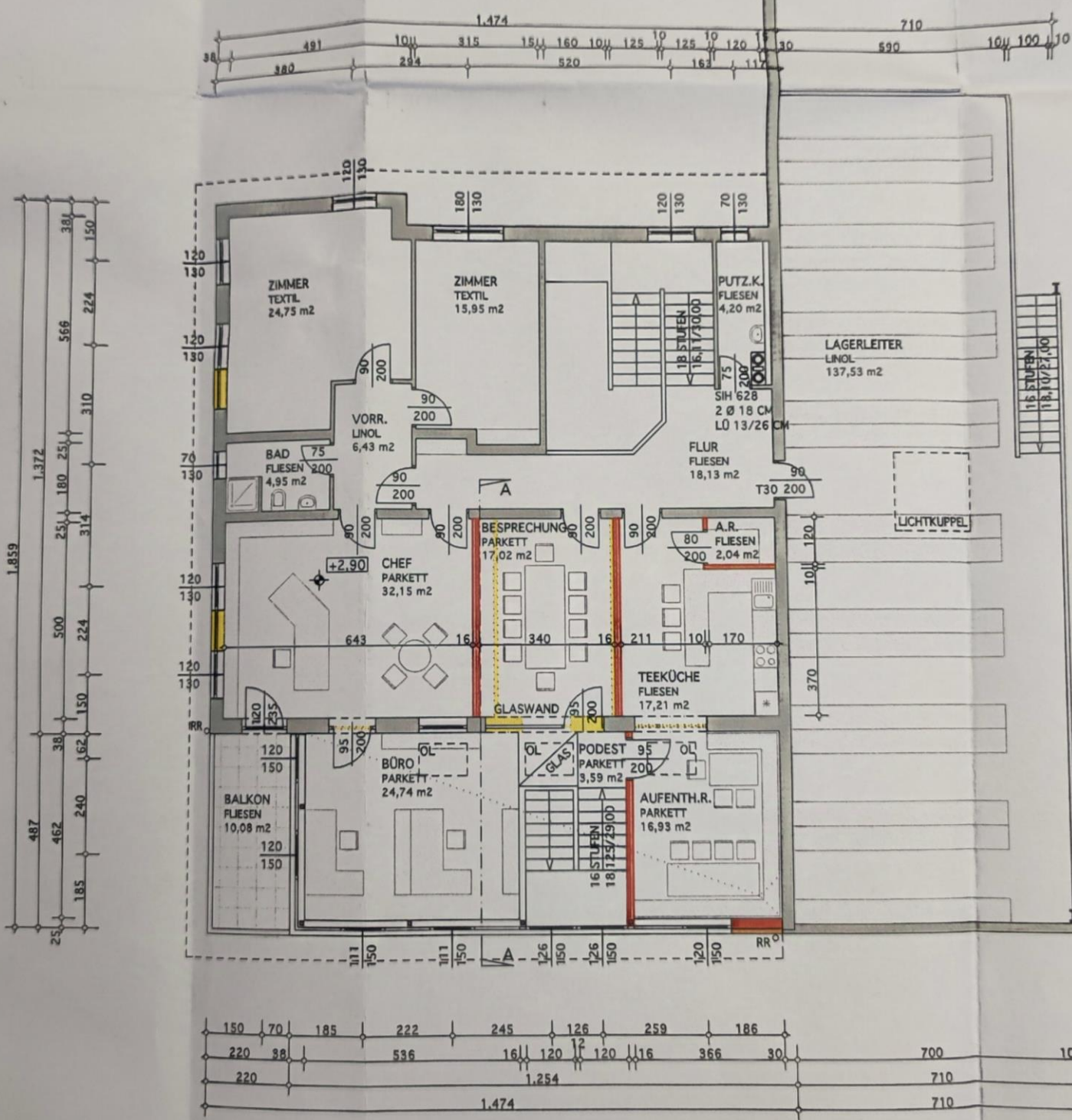
GRUNDRISS OBERGESCHOSS
