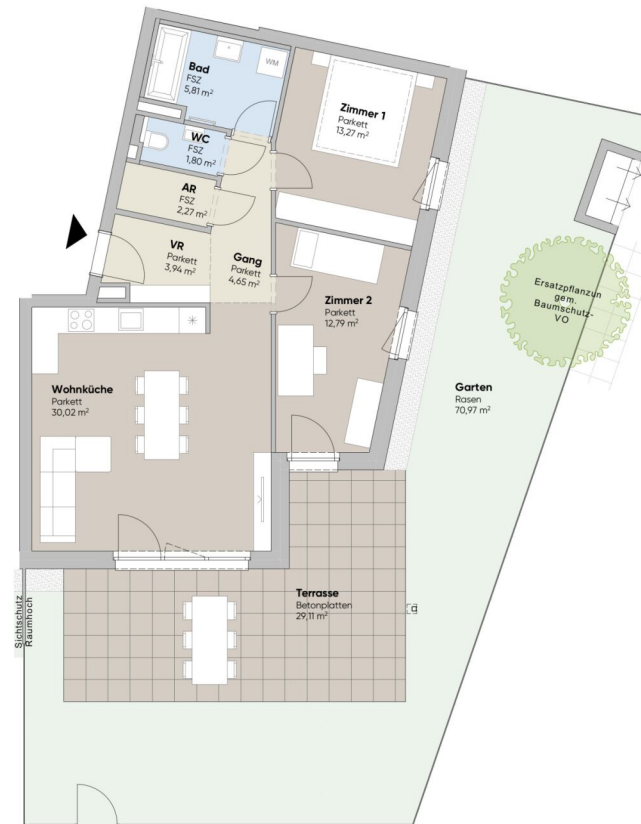
Erdgeschoß
