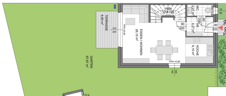
Erdgeschoss
