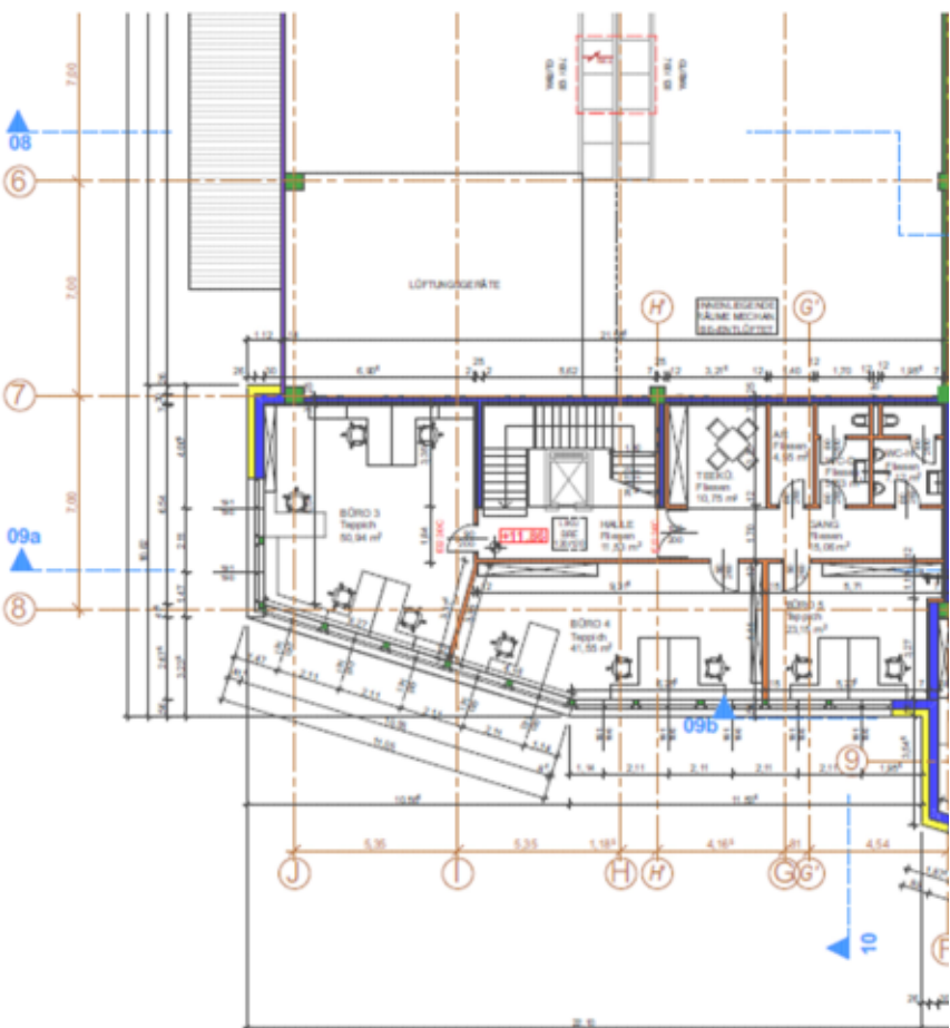
2.OBERGESCHOSS HALLE 4 (Objekt 18)
