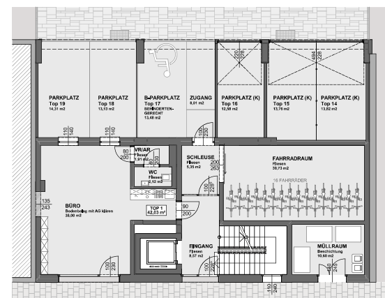
ERDGESCHOSS
