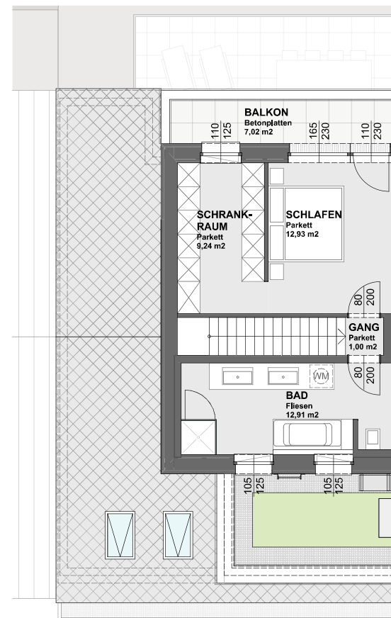
TOP 12 - 2. DACHGESCHOSS
