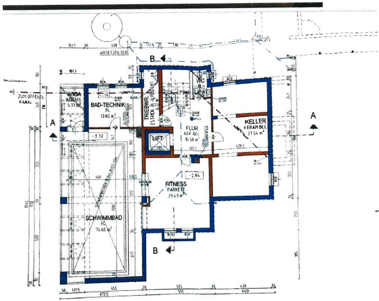
UNTERGESCHOSS
