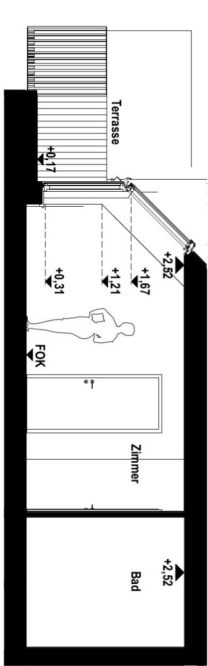
Schnitt
