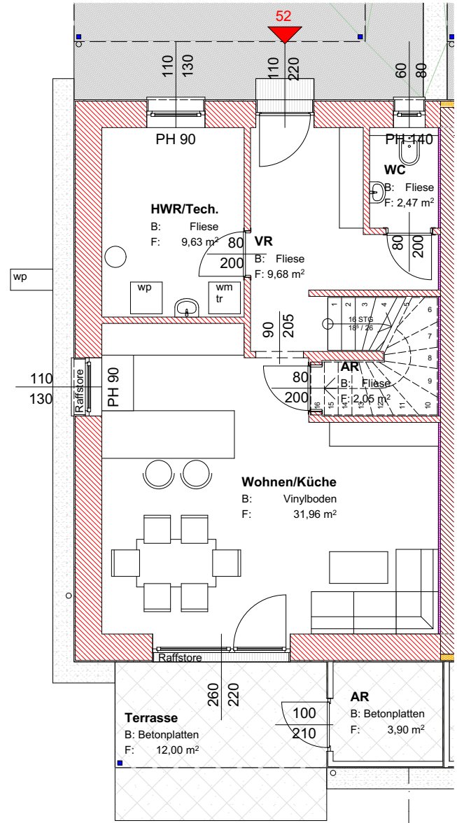
0. Erdgeschoss 1:100
