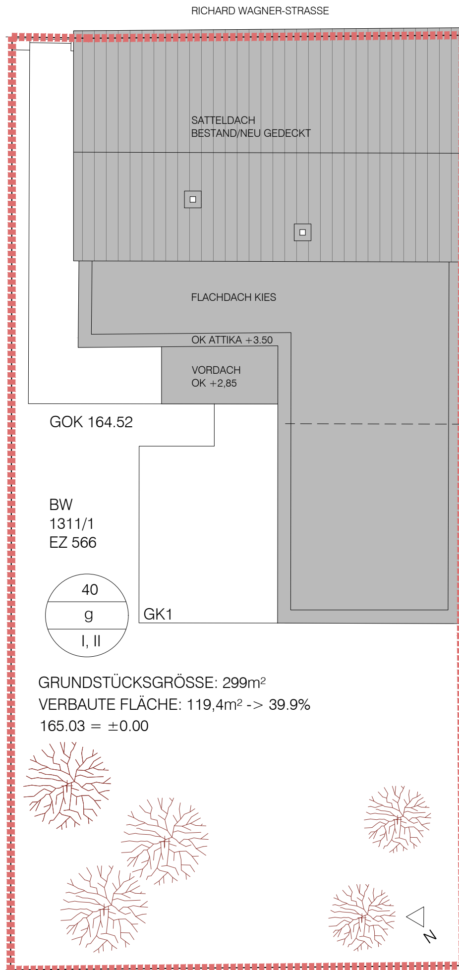
DACHAUFSICHT
