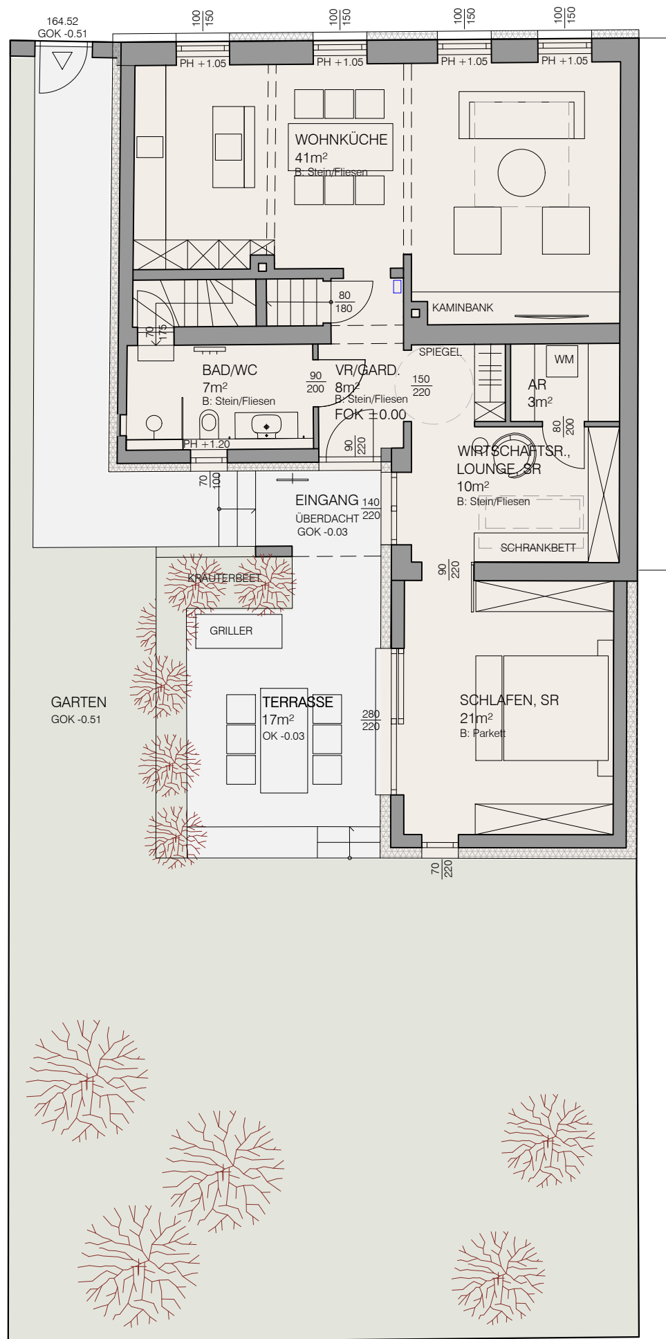
GRUNDRISS
