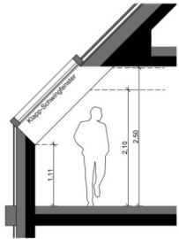
Schnitt 1
