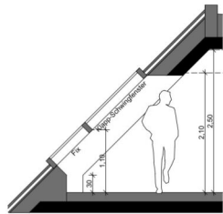
Schnitt 1
