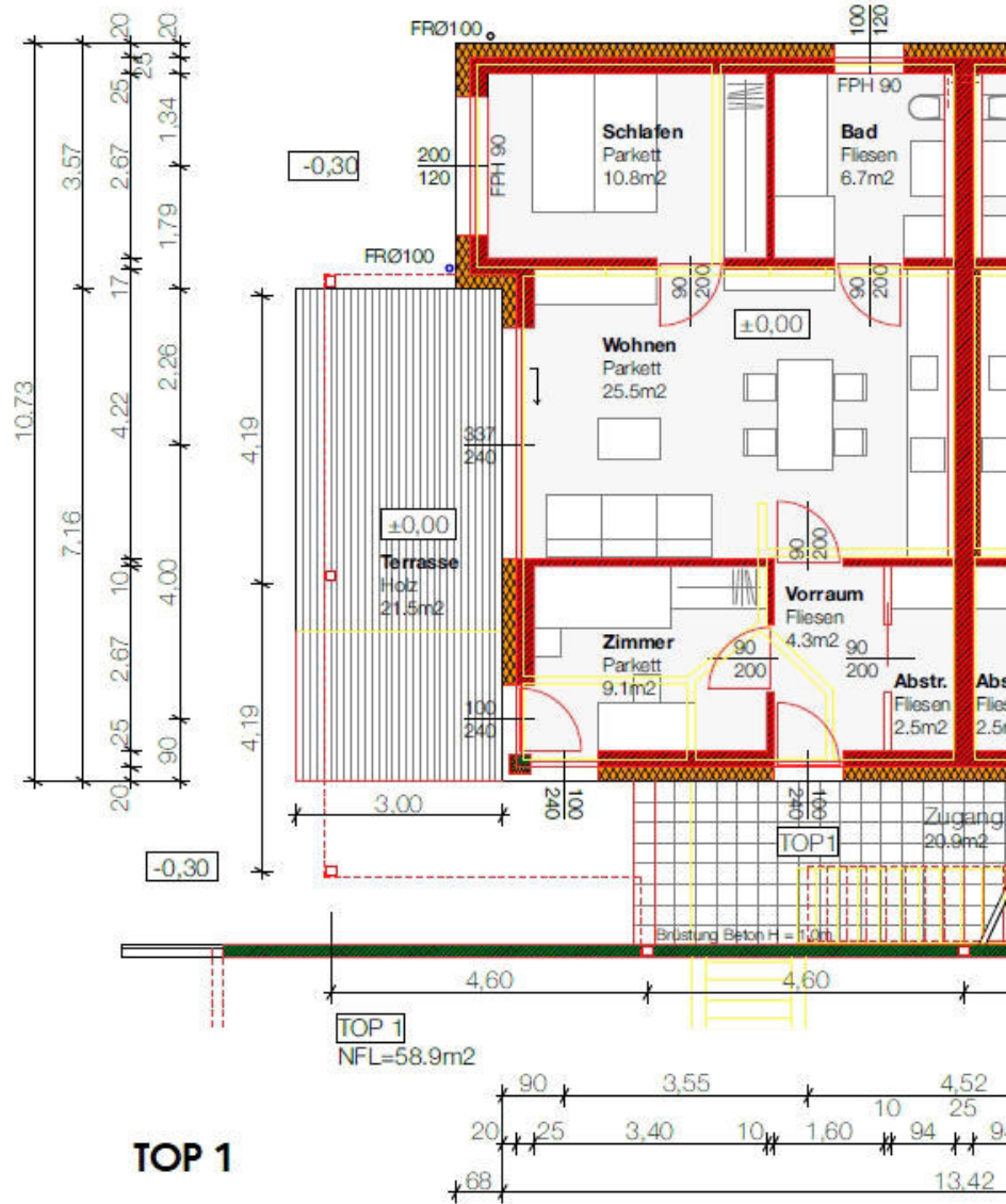
GRUNDRISS ERDGESCHOSS
