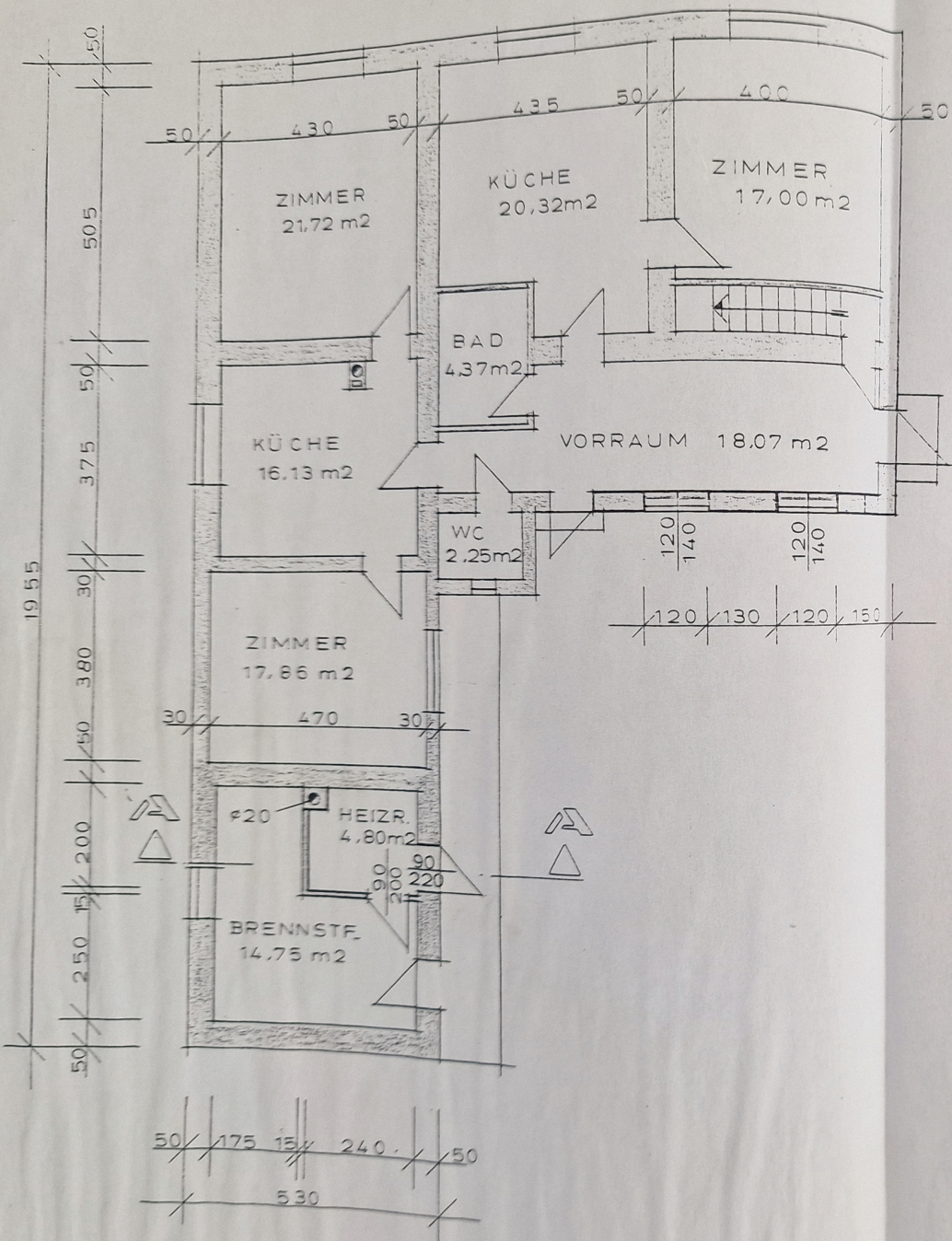
GRUNDRISS
