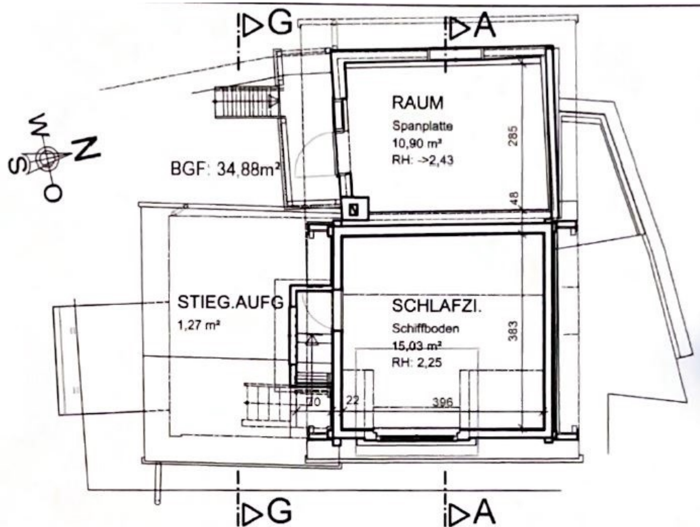
Grundriss Dachgeschoß
