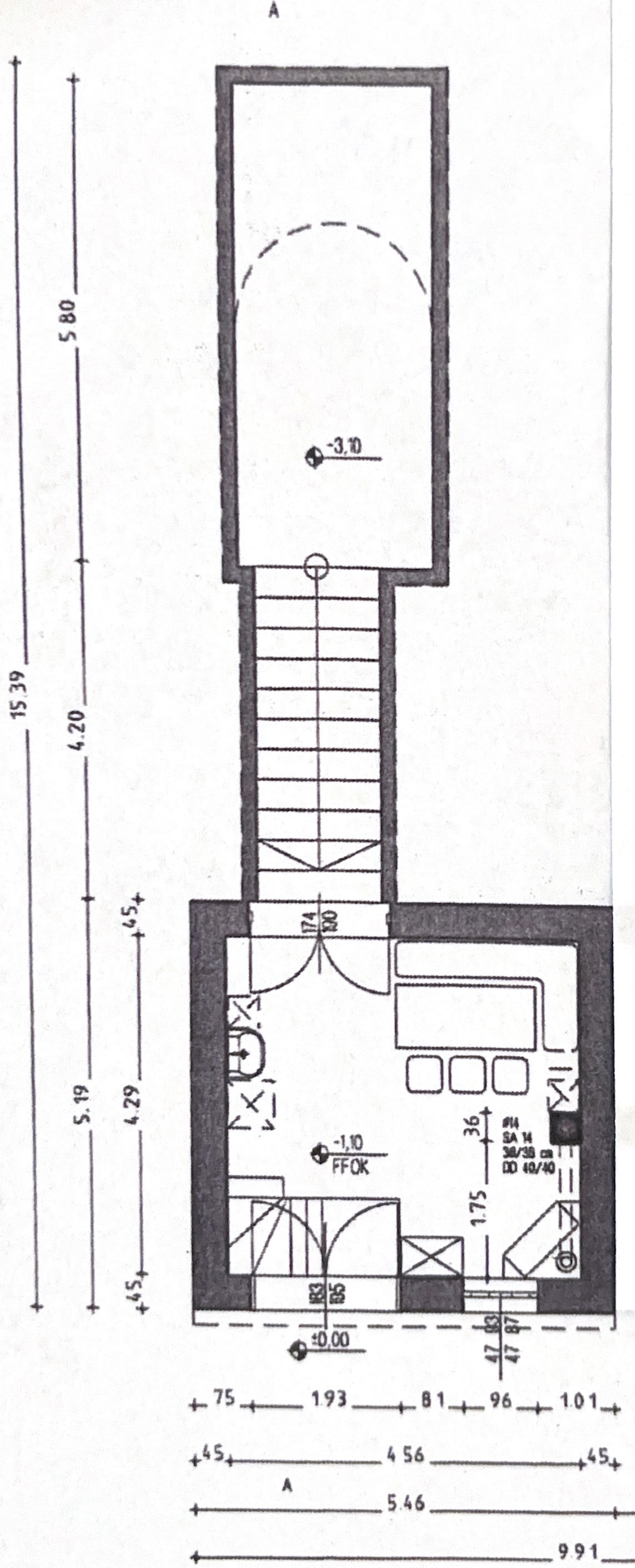
GRUNDRISS M 1:100
