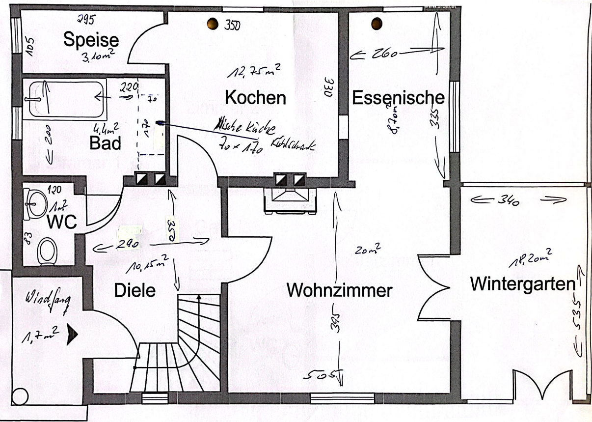
Skizze Erdgeschoss
