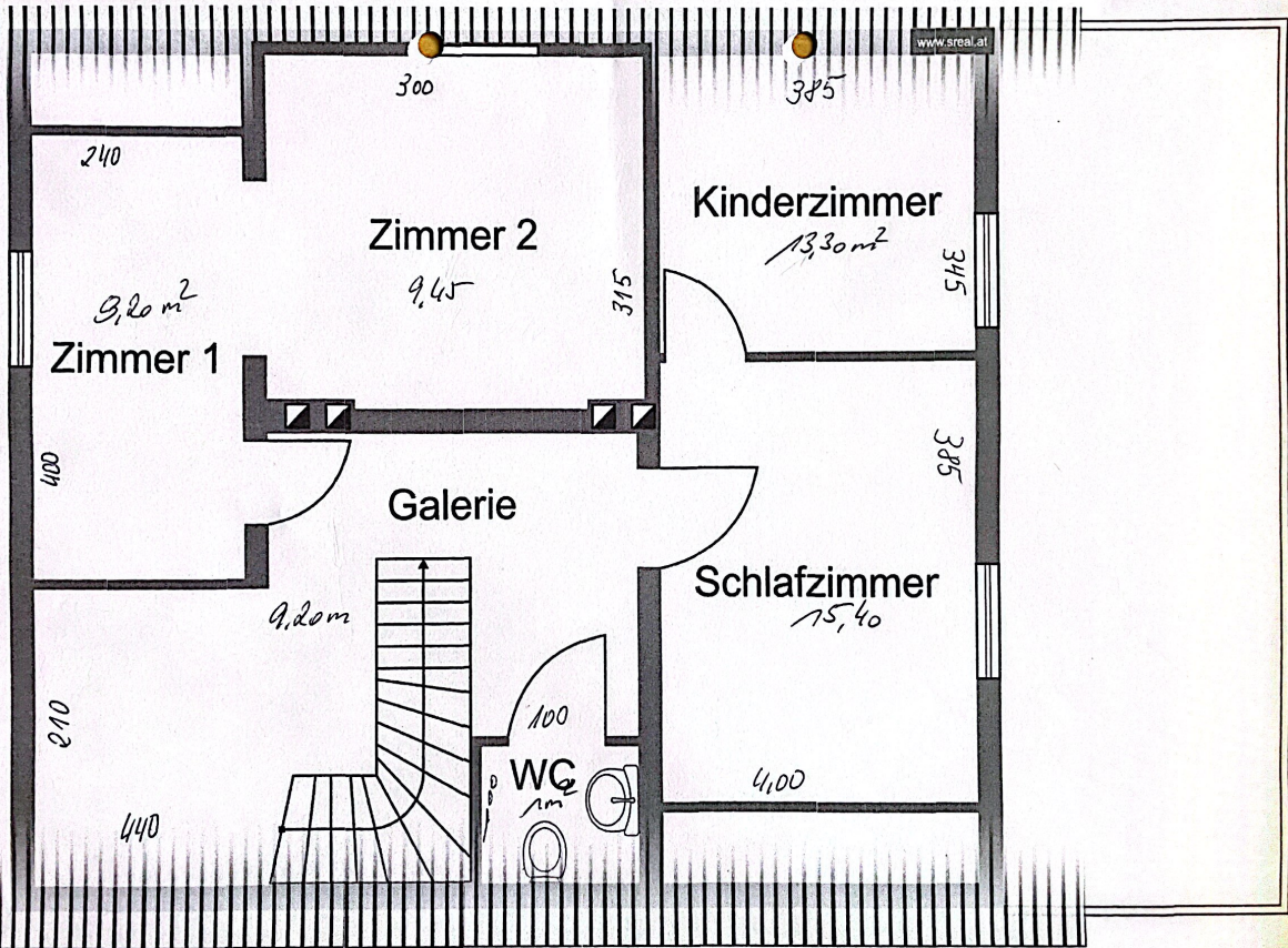
Skizze Dachgeschoss
