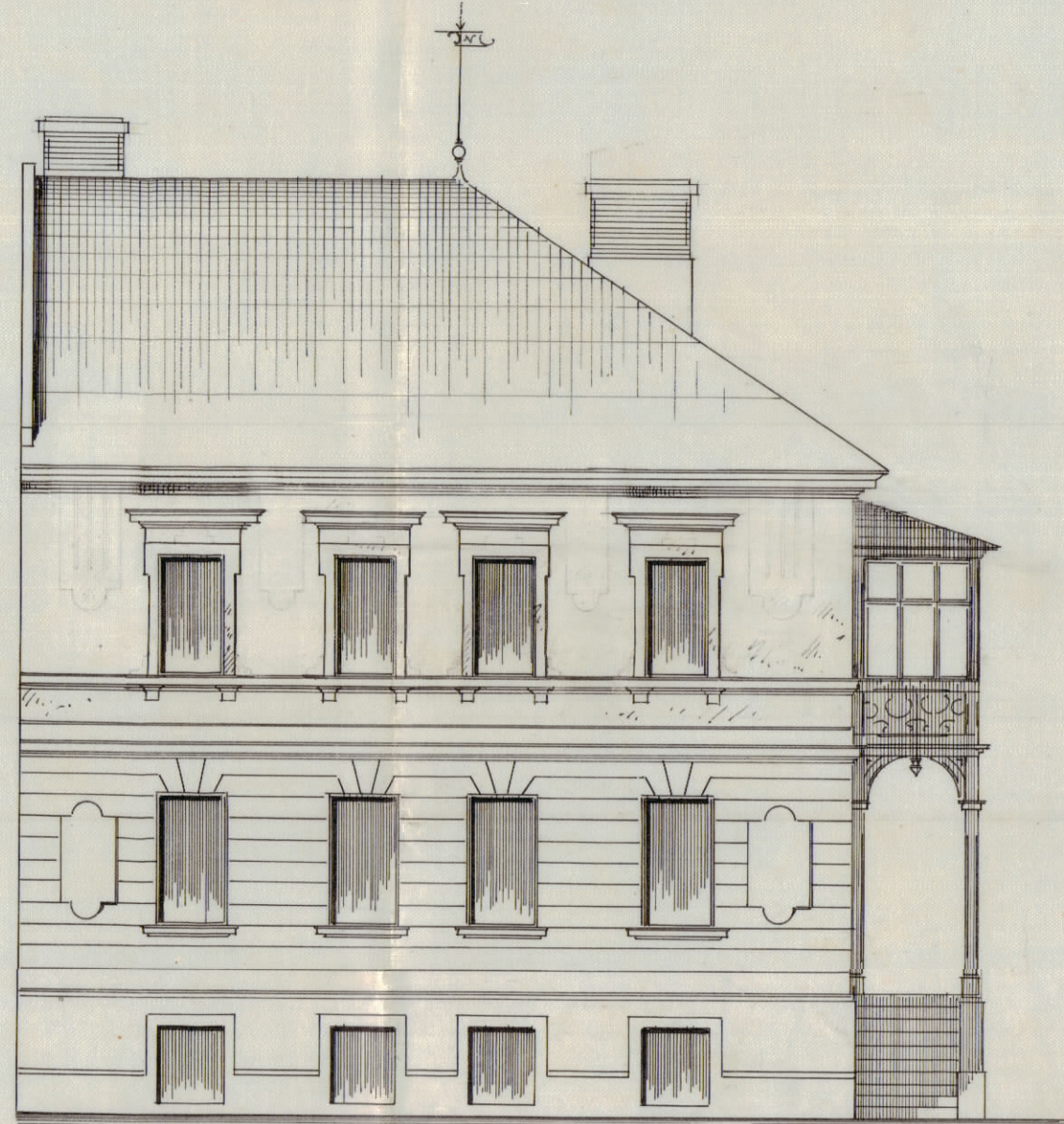
Vorderansicht.
