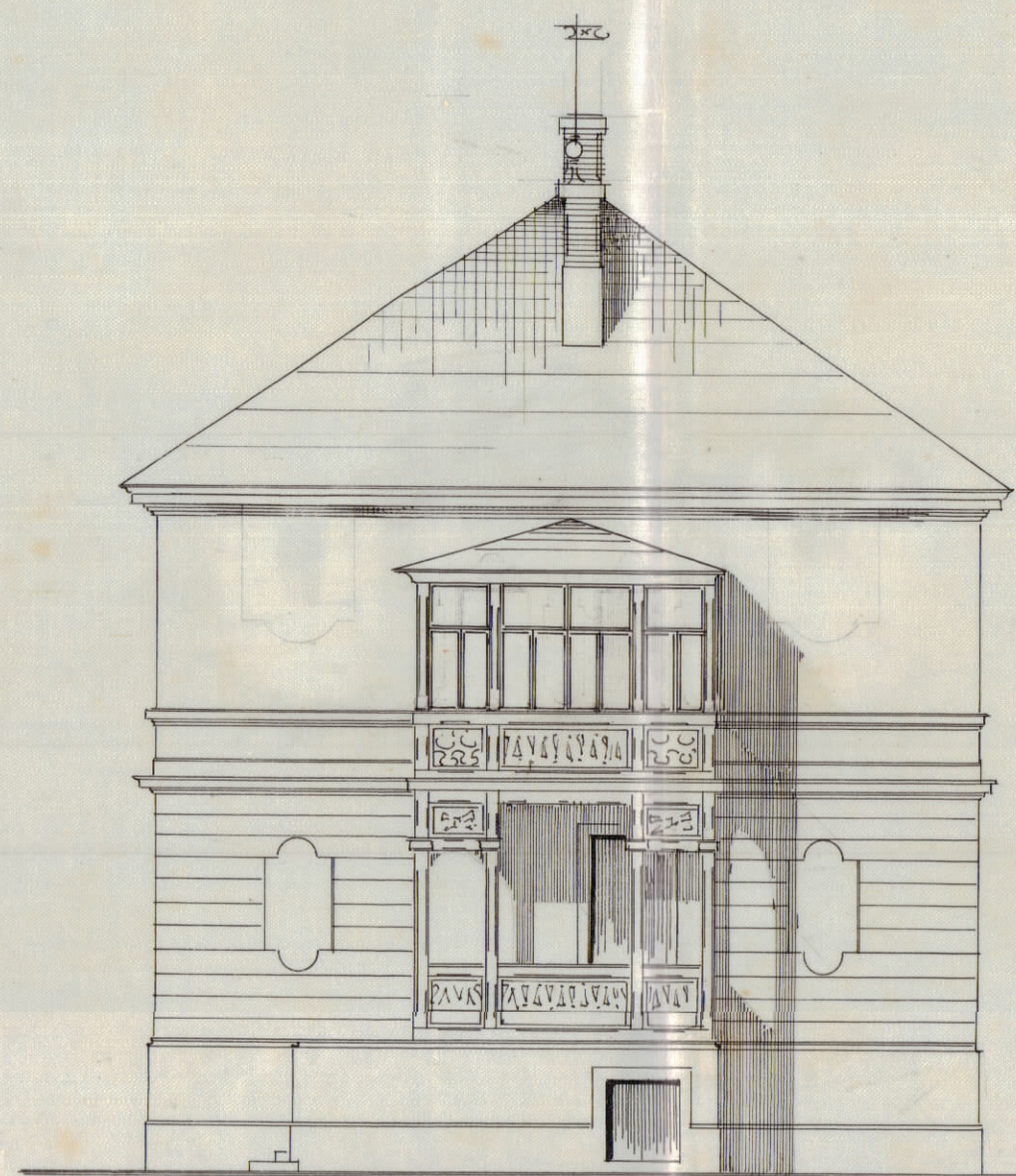
Seitenansicht.
