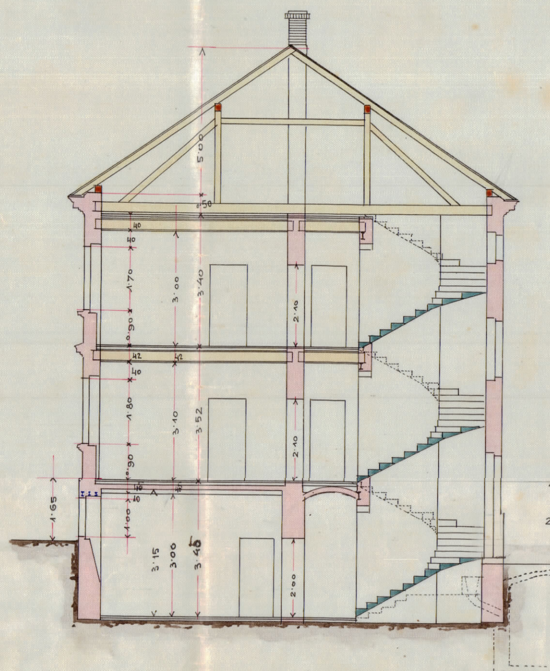
Querschnitt.
