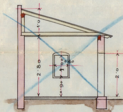
Profil
