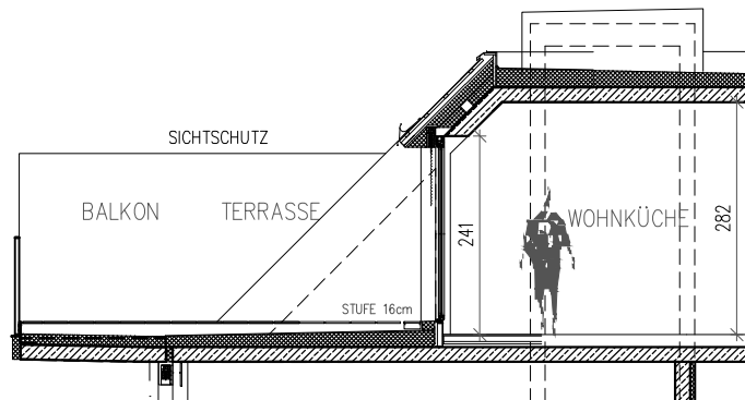
SCHNITT A
