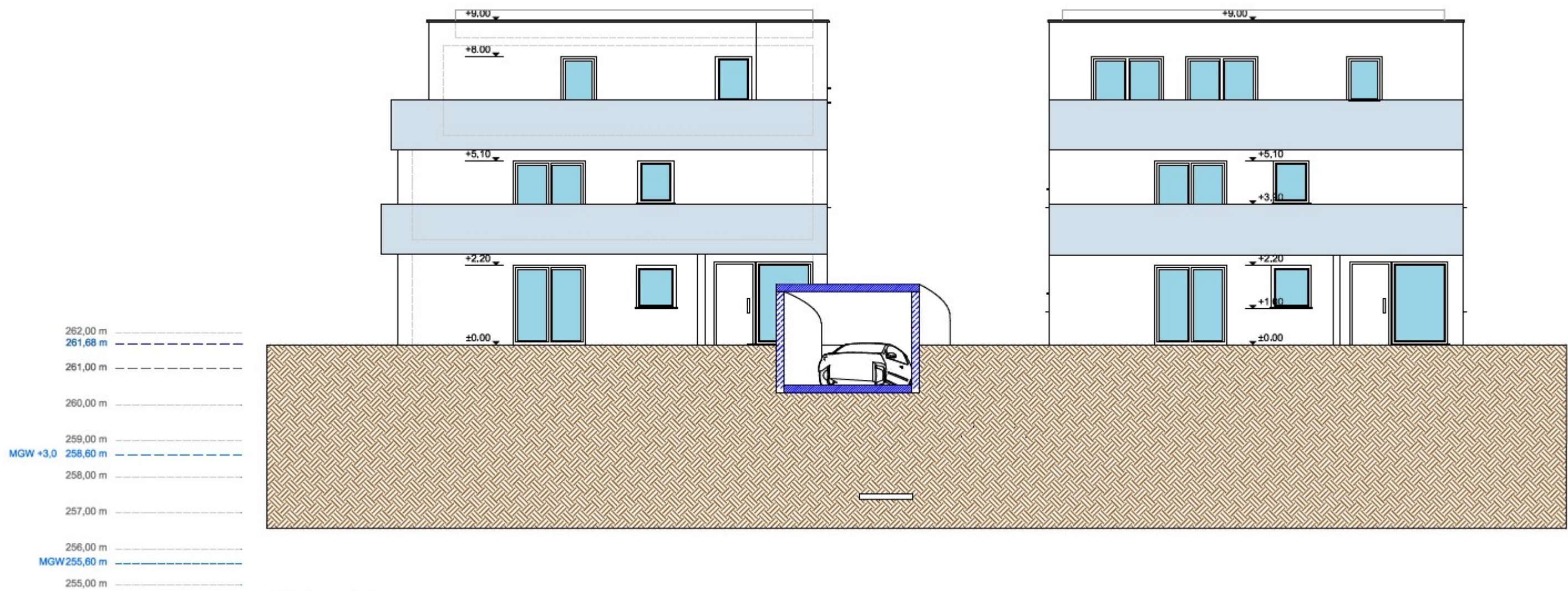
Südansicht
