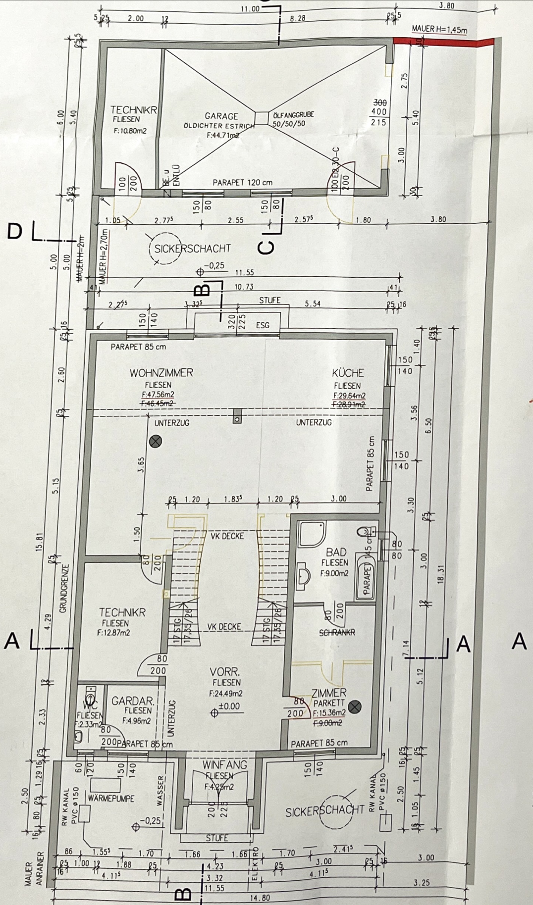
GRUNDRISS ERDGESCHOSS
