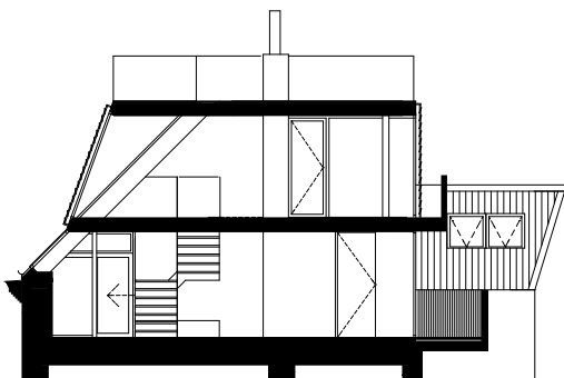
SCHNITT
