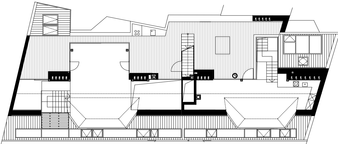
2. DACHGESCHOSS
