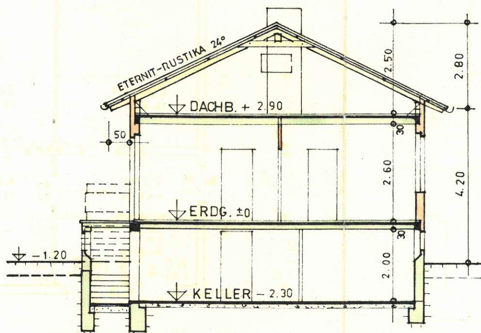
SCHNITT A-B
