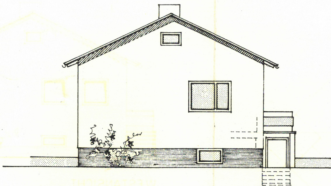
OSTANSICHT
