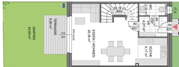
Erdgeschoß
