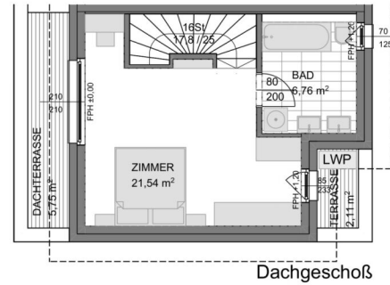
Dachgeschoss
