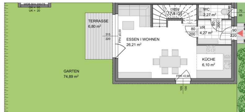
Erdgeschoß
