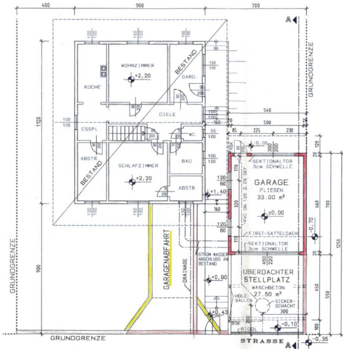
GRUNDRISS: GARAGE
