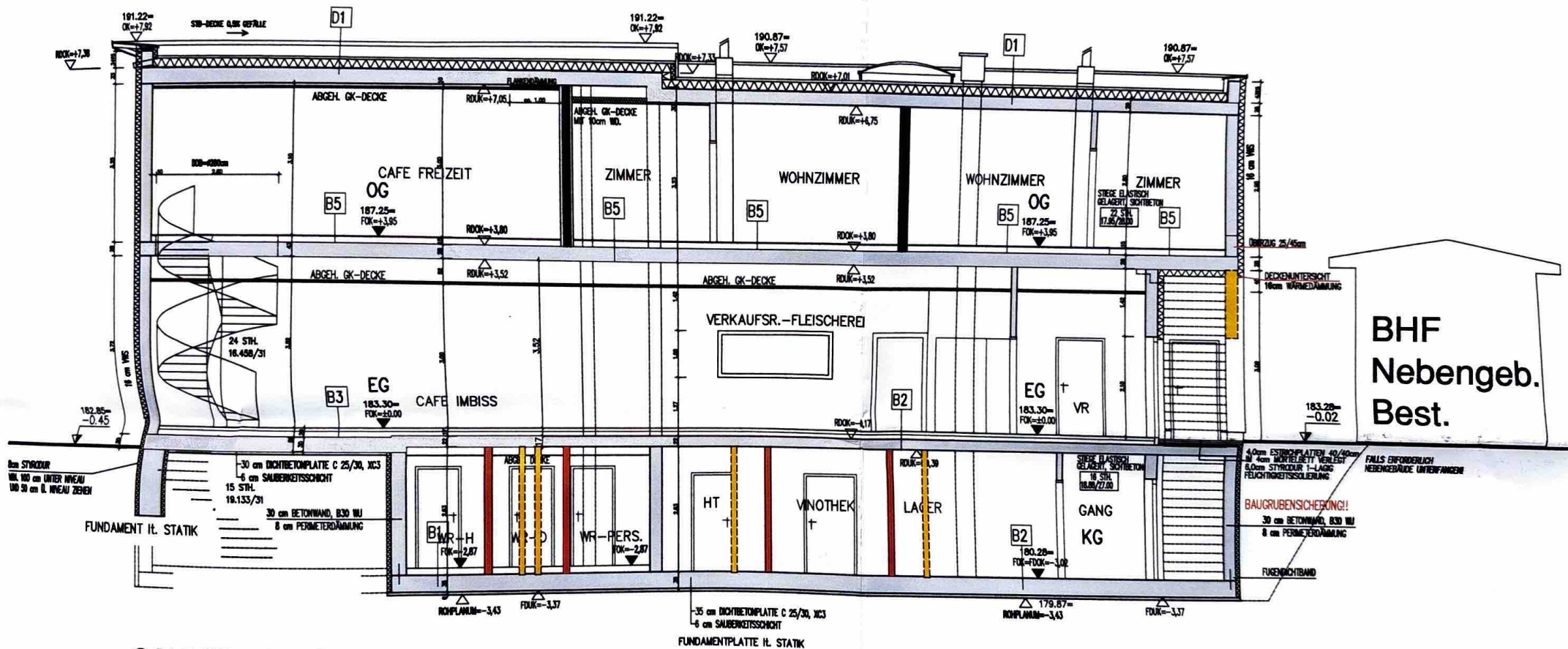
SCHNITT B-B
