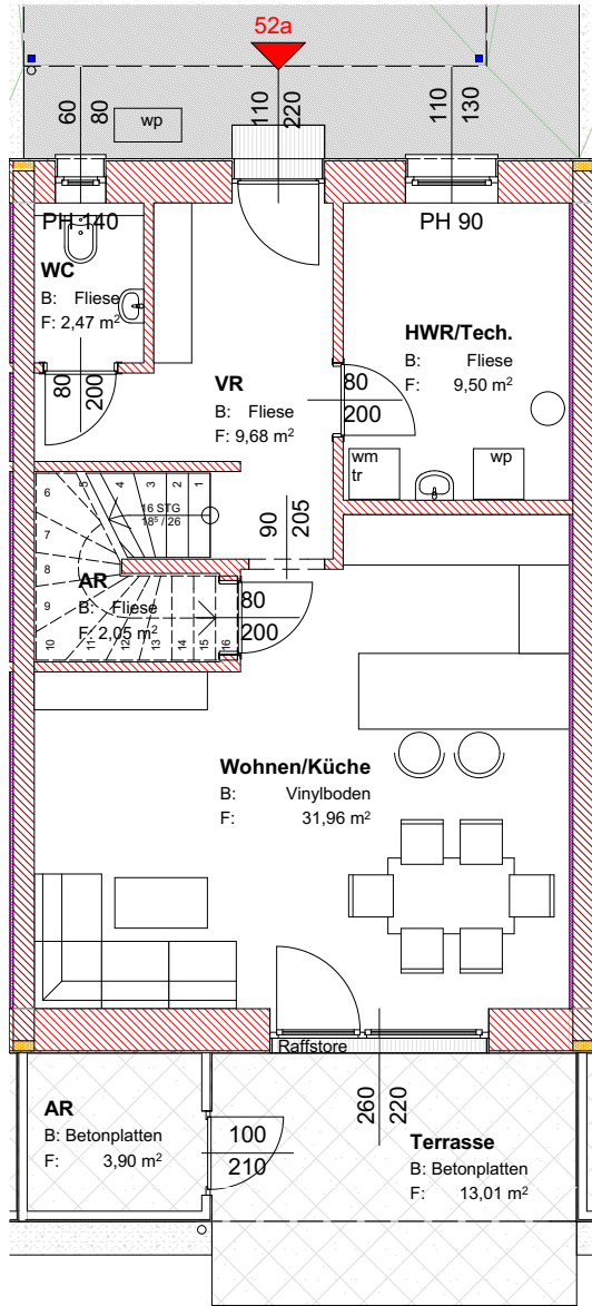
0. Erdgeschoss 1:100
